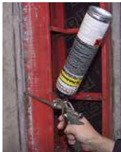
Dosierpistole aus rostfreiem Metall, mit Teflonbeschichtung
